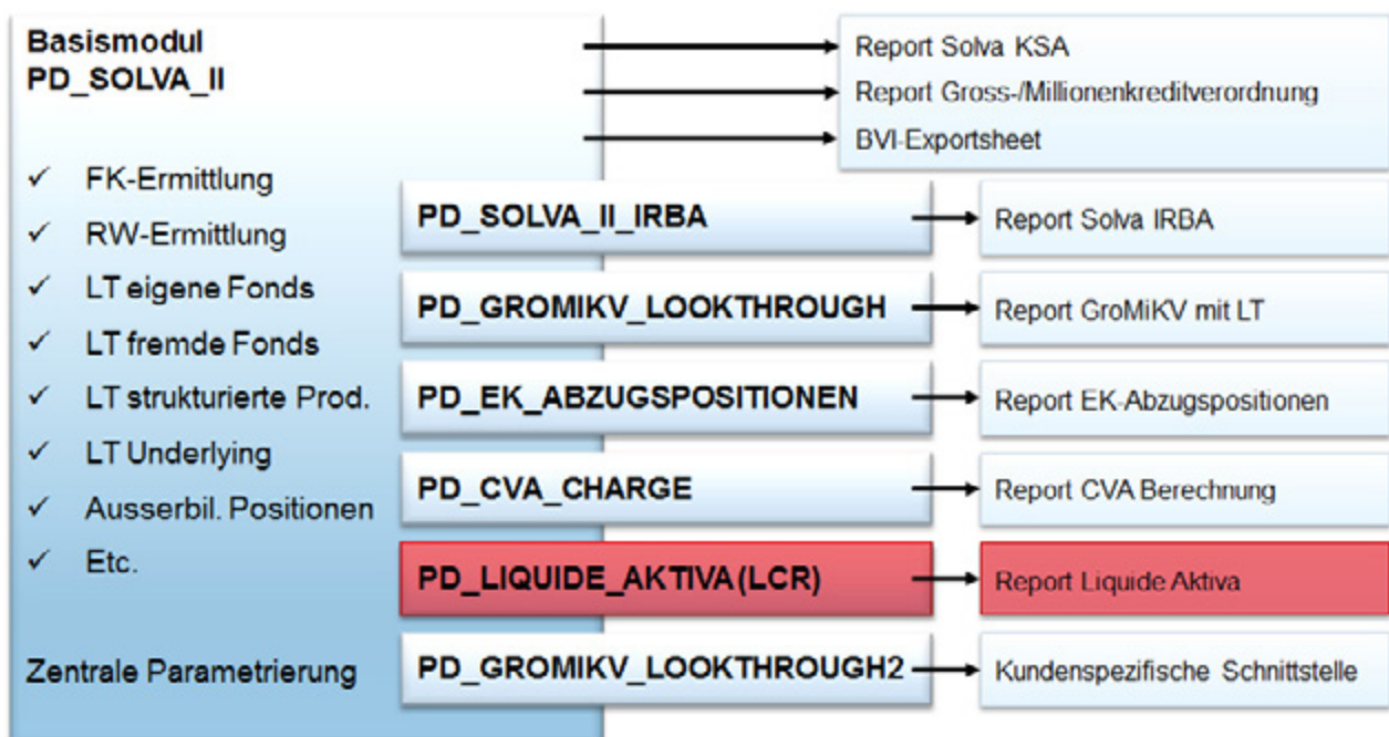
Abb. 2: Solvabilitätsmeldungen nach CRD IV in XENTIS
